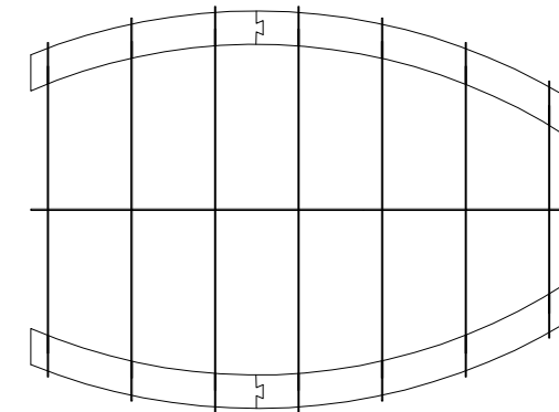
Planta 2 Riostra R2
