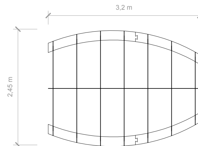
Planta 1 Riostra R5
